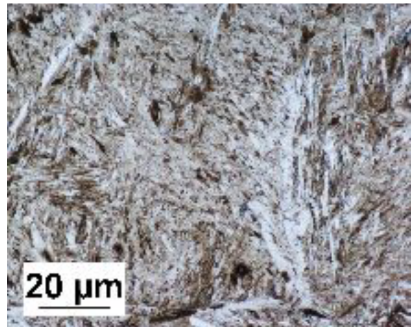
(d) Txz-100x cross section
